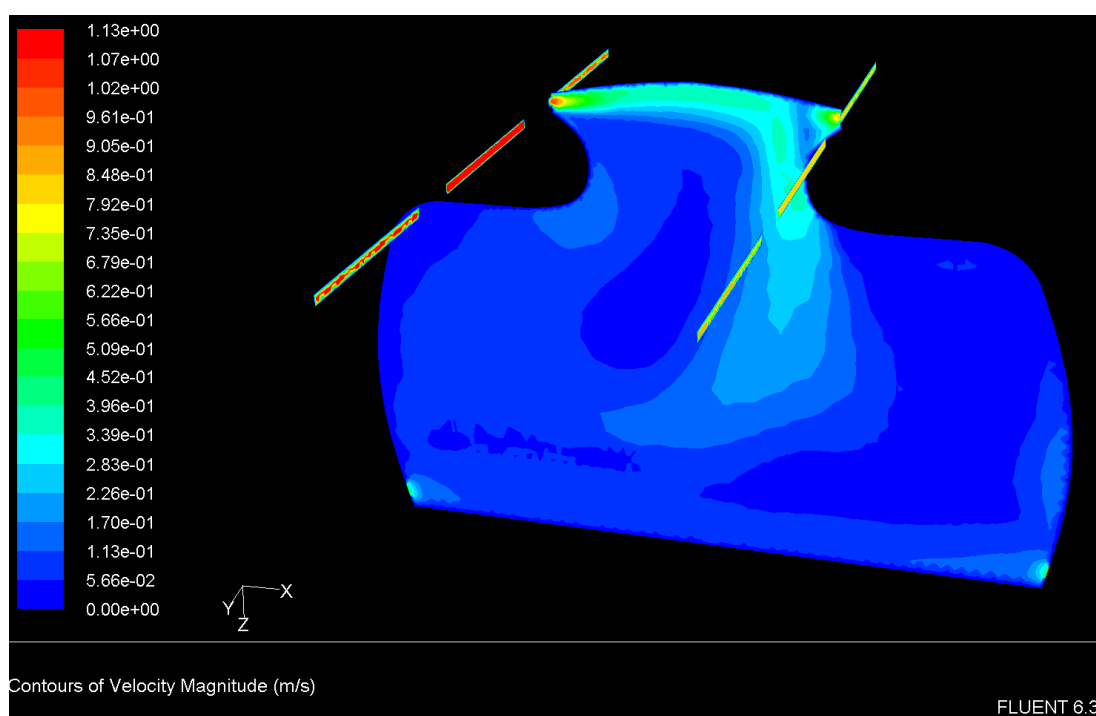
Figura 19: Escoamento na cabine: entradas de ar e fluxo de velocidades em um plano
