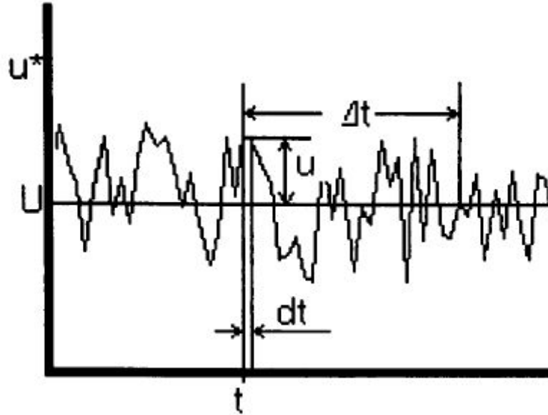
Figura 8: Componente da velocidade turbulenta instantânea com relação ao tempo
